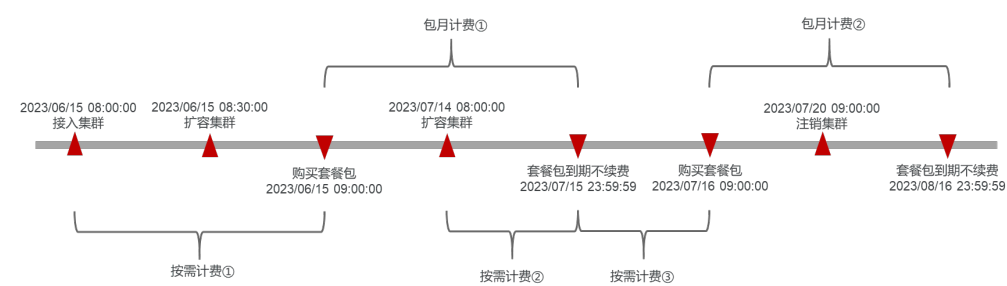
图 4-4 计费构成轴
