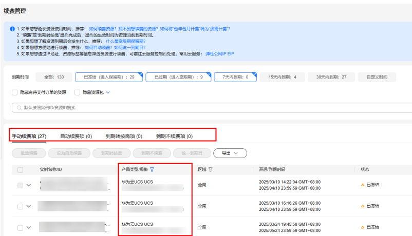
图 5-6 续费管理
